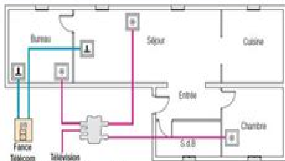
Installation traditionnelle
